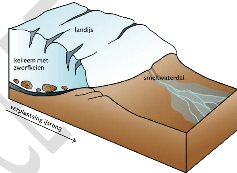
Fig. x. Schematische weergave van het schuivende landijs dat gedurende de één na laatste ijstijd allerlei materiaal vanuit het noorden hiernaartoe bracht. Gemaakt door S. van den Wittenboer.
